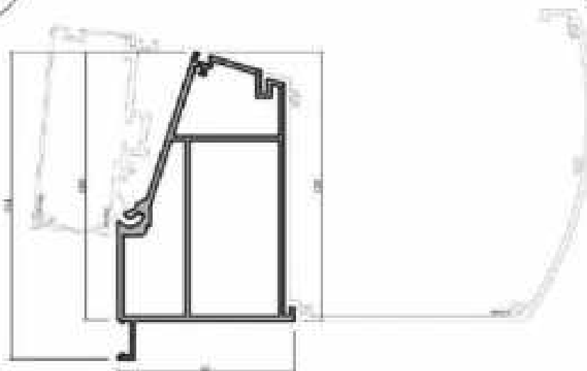
880.2101 ( 3,438 kg/ml ) GRAIN 121 (20R) PROFIL
