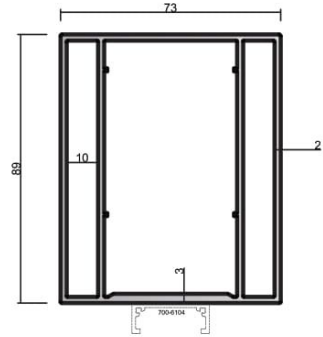
580-1201 ( 2,743 kg/mt ) SRA150 M03 TAŞIYICI DİKME PROFİLİ
