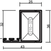
580-4201 ( 0,613 kg/mt ) SRA150 V02 KANAT PROFİLİ
