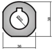
580-6101 ( 2,286 kg/mt ) SRA140 HAREKET AKTARMA PROFİLİ
