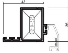
580-4202 ( 0,683 kg/mt ) SRA150 KANAT PROFİLİ
