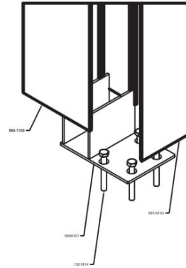
DETAJ 05 ALT MONTAJ
