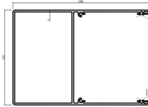
580-1103 ( 4,099 kg/mt ) TAŞIYICI DİKME PROFİLİ
