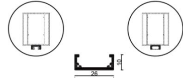
580-1201 ( 2,743 kg/mt ) SRA150 M03 TAŞIYICI DİKME PROFİLİ
